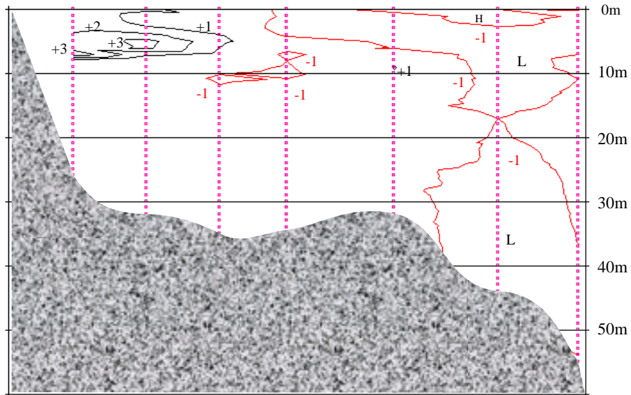
7月26日-14日 水温変化鉛直断面図
