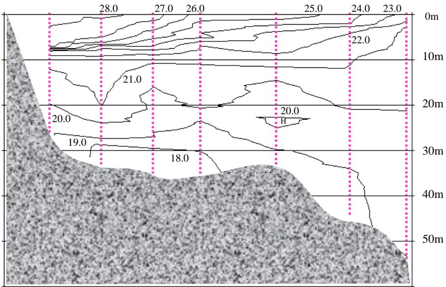
7月26日 水温鉛直断面図
