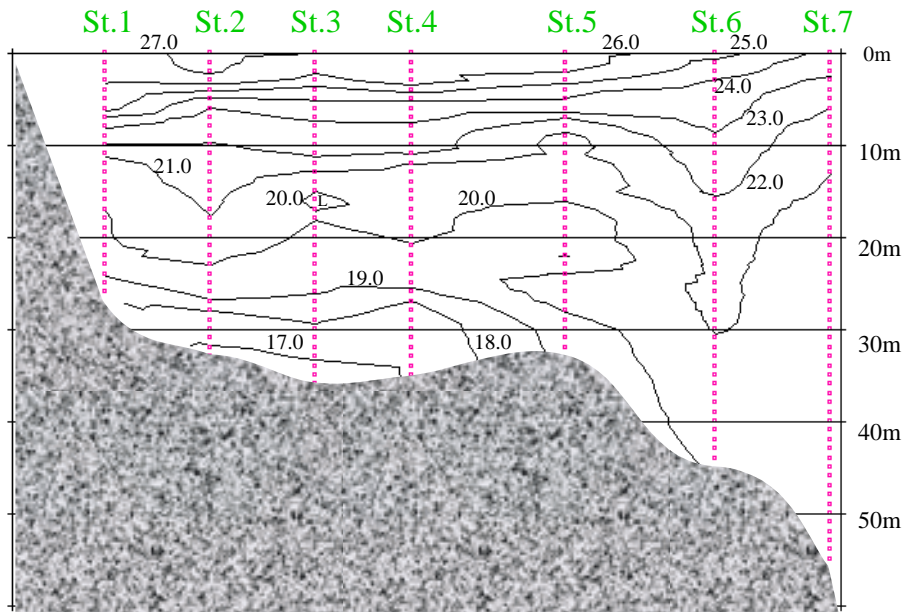
7月14日 水温鉛直断面図
