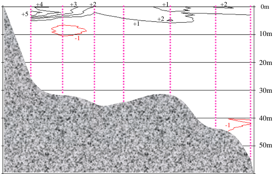
8月22日-11日 塩分変化鉛直断面図
