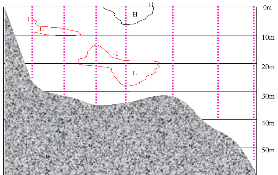
10月27日-13日 塩分変化鉛直断面図
