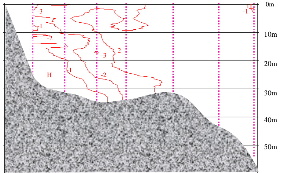
11月27日-13日 水温変化鉛直断面図
