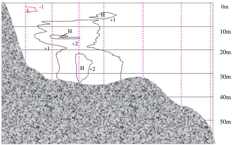
平成13年 4月23日-17日 水温変化鉛直断面図
