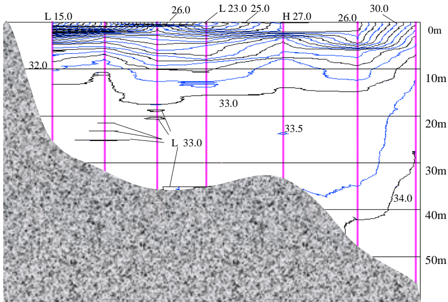
平成13年6月26日 塩分鉛直断面図
