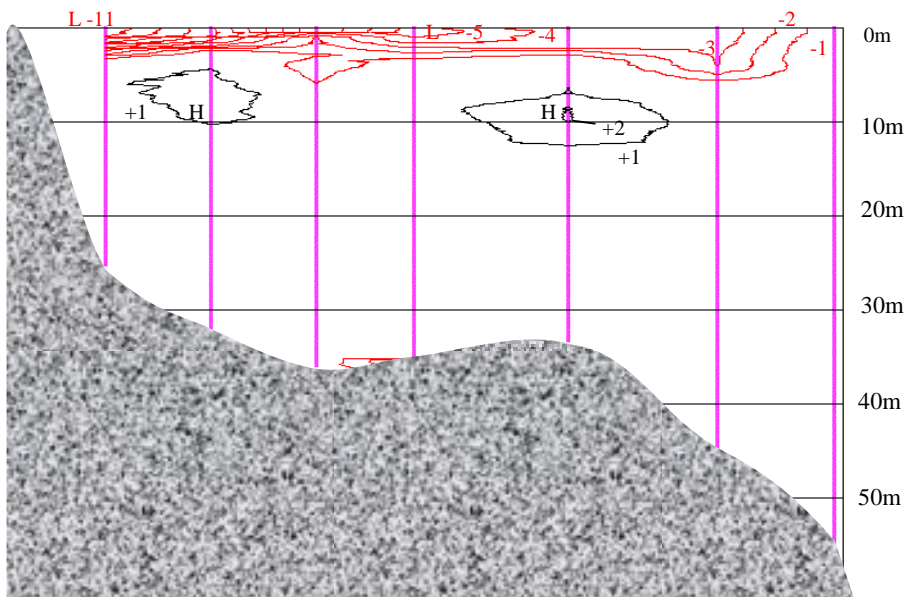
平成13年 6月26日-12日 塩分変化鉛直断面図
