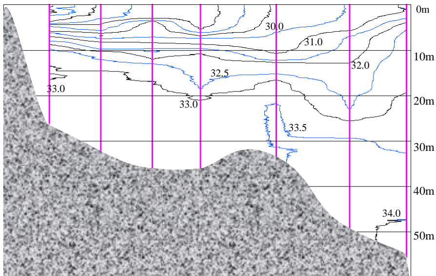
平成13年6月12日 塩分鉛直断面図
