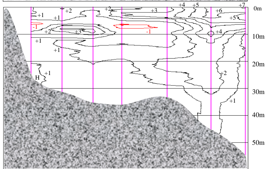
平成13年 7月25日-10日 水温変化鉛直断面図
