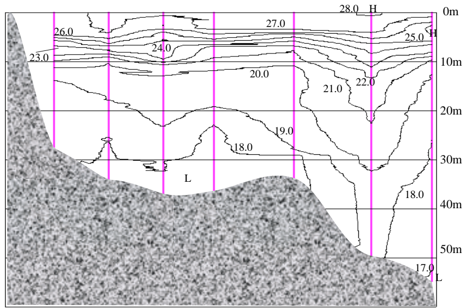
平成13年7月25日 水温鉛直断面図
