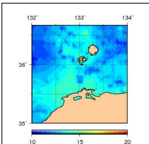
隠岐海峡周辺海域
