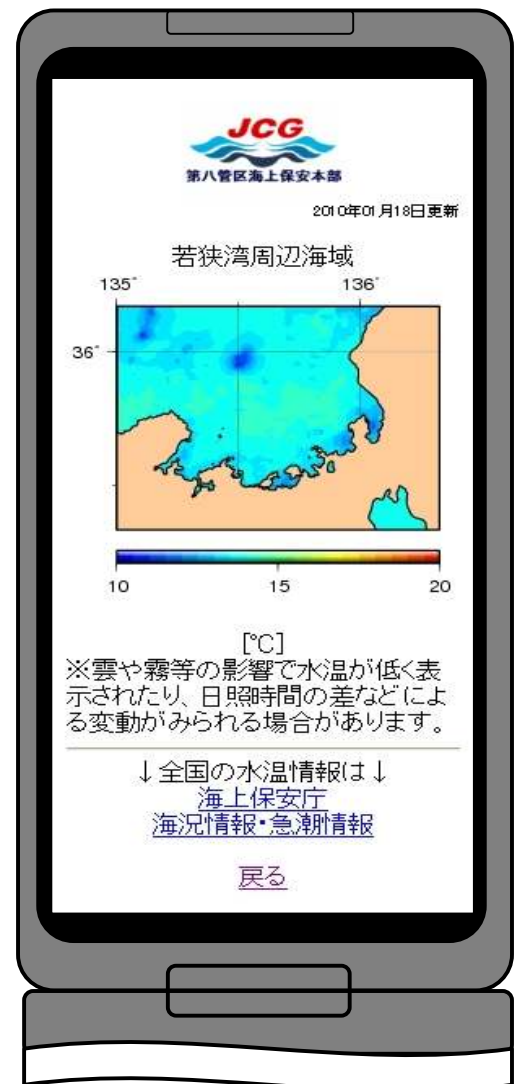
若狭湾周辺海域
