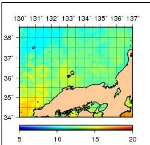
八管区周辺海域
