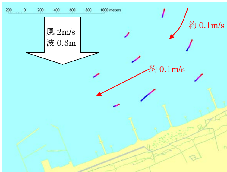
図3-3 (6月3日 調査海域全域)
