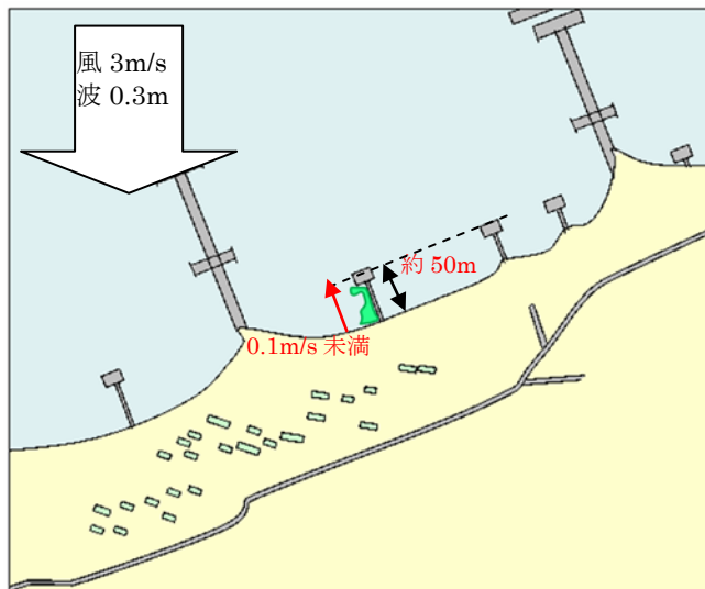
図6-1 (6月2日 調査海域全域)
