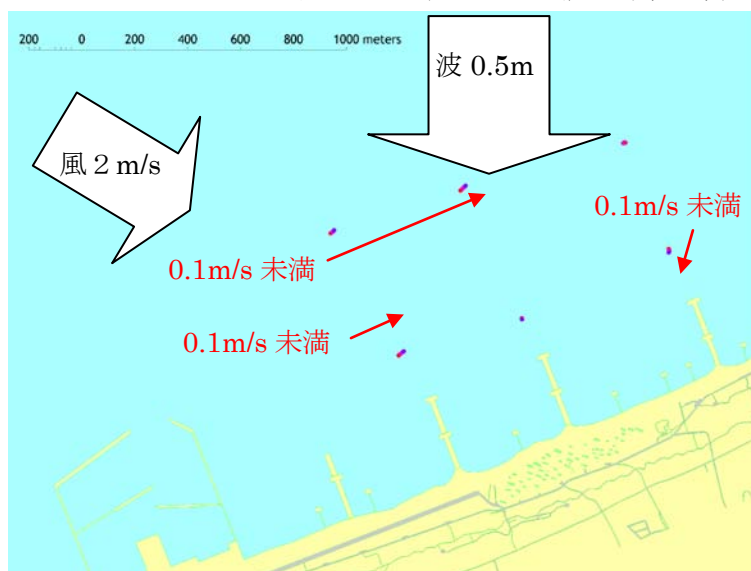
図3-1 (6月1日 調査海域全域)
