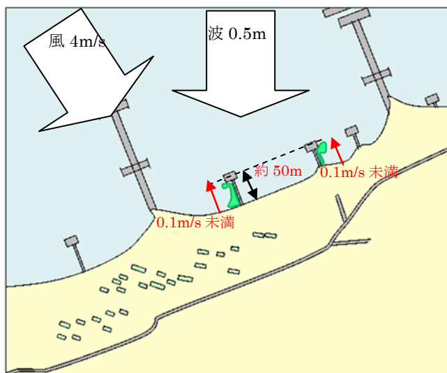
図6-1 (6月2日 調査海域全域)
