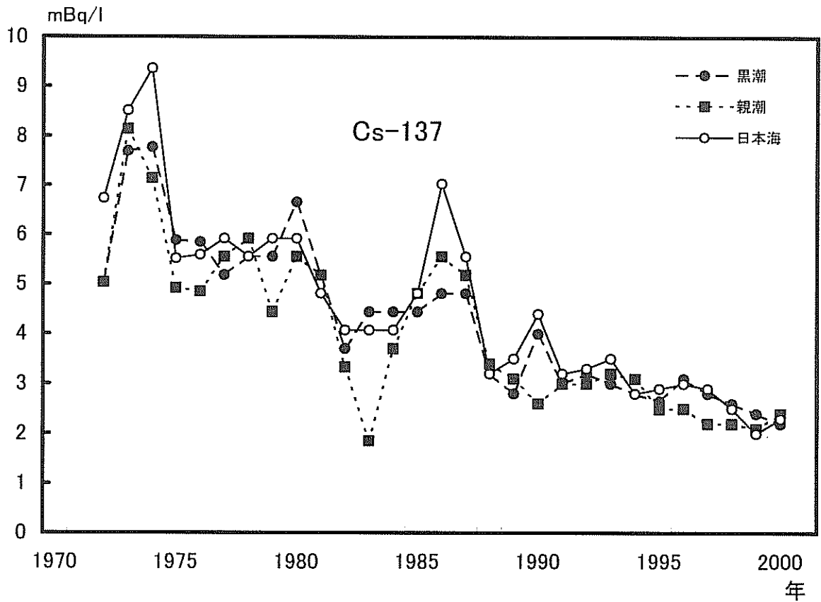
図1-2 日本近海海水中のSr-90, Cs-137の年平均濃度の経年変化
