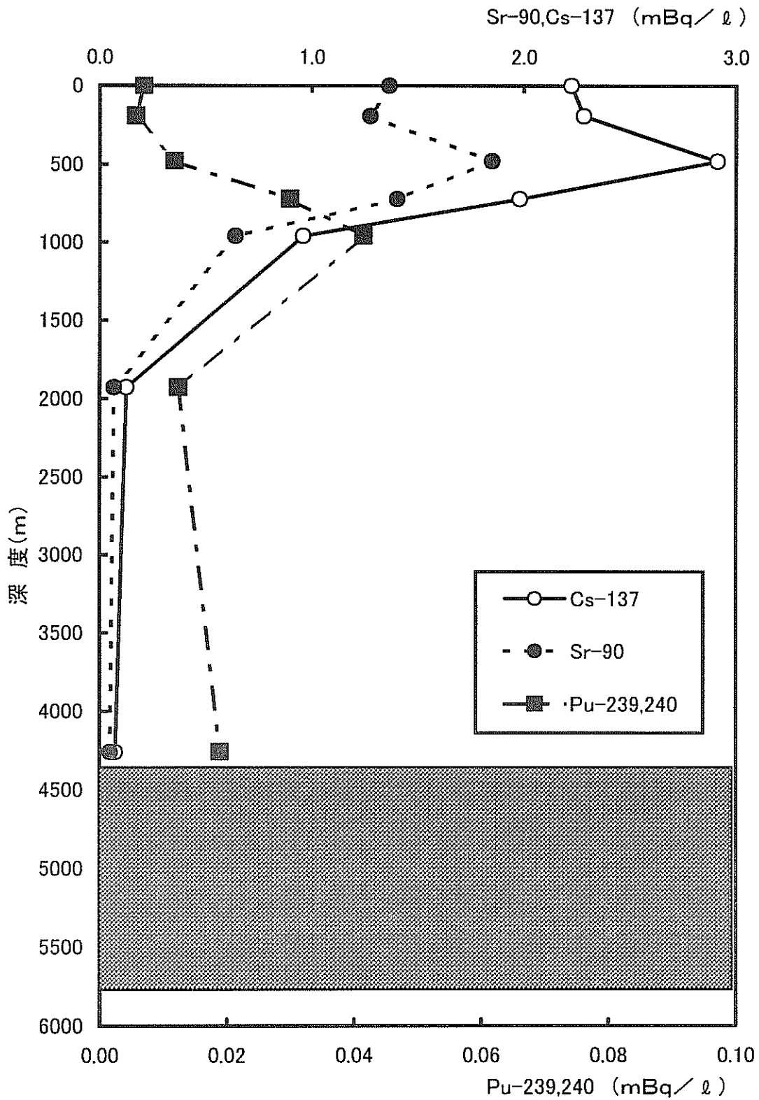
図3-2 測点Aにおける海水中の各核種の鉛直分布
