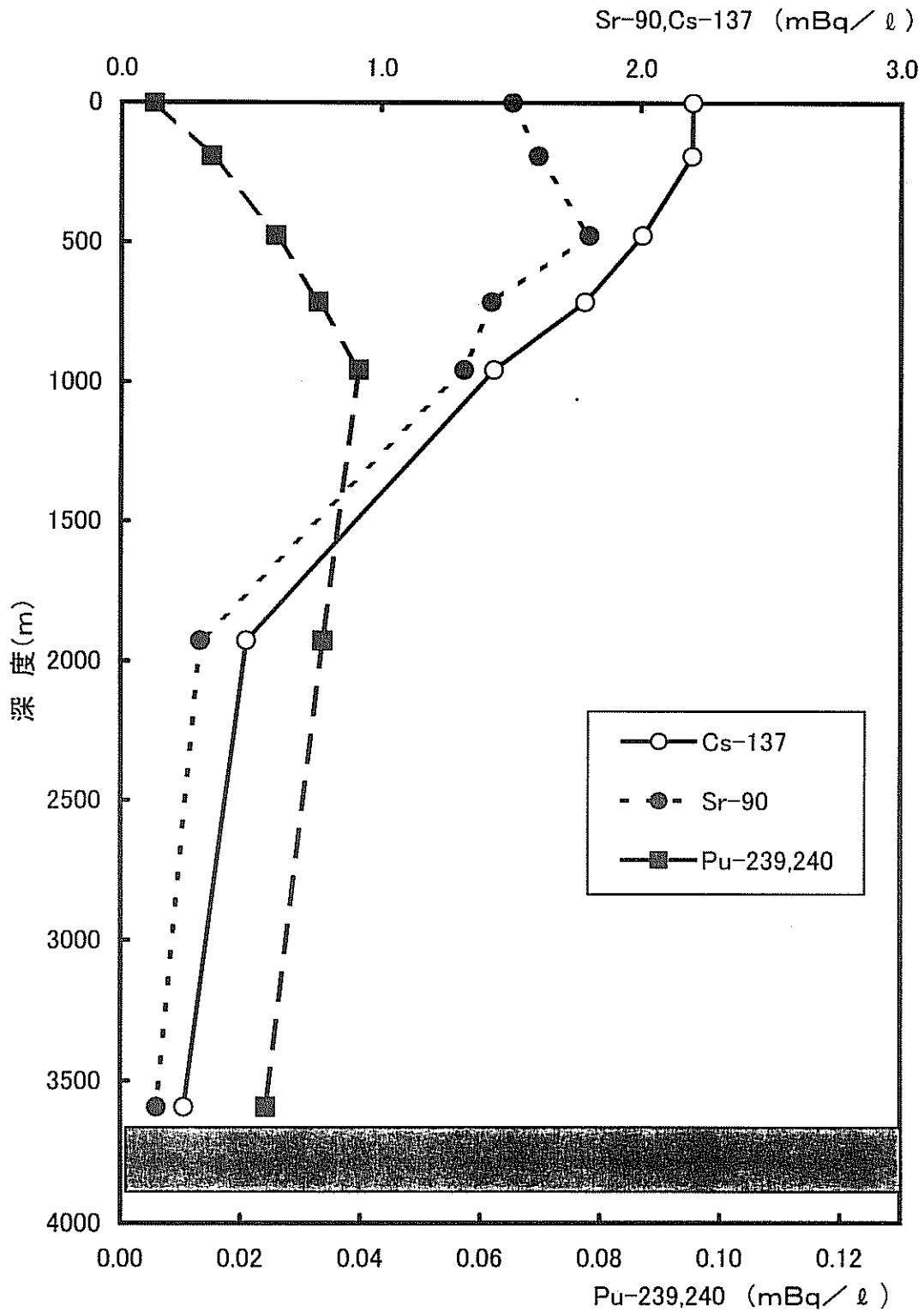
図3-10 測点NO-7における海水中的の各核種の鉛直分布
