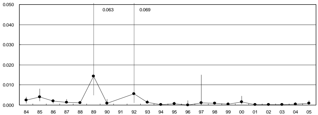
水銀(Mercury) (WESTPAC Area 0m)
