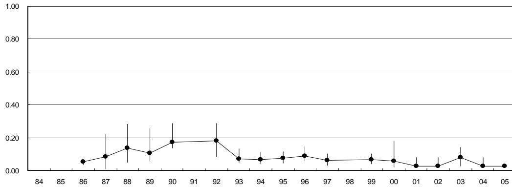
油分(Petroleum Oil) (WESTPAC Area 0m)
