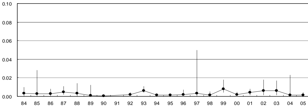
水銀(Mercury) (WESTPAC Area 0m)
