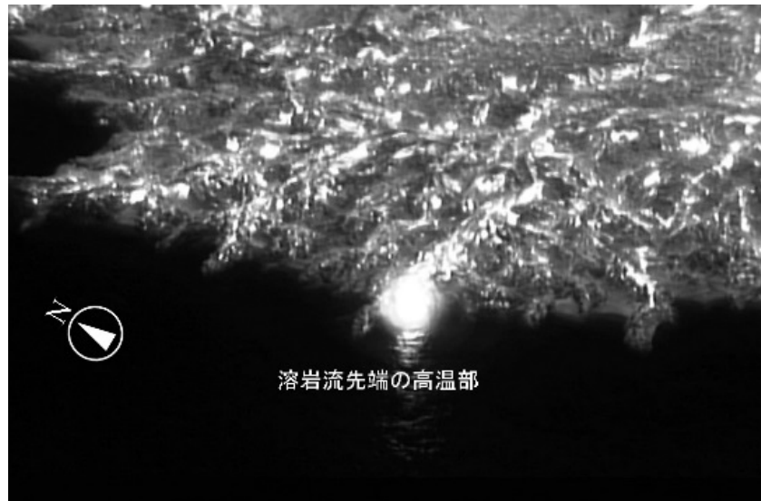
図2 熱画像（溶岩流先端の白色蒸気と高温部）（8月11日撮影）
