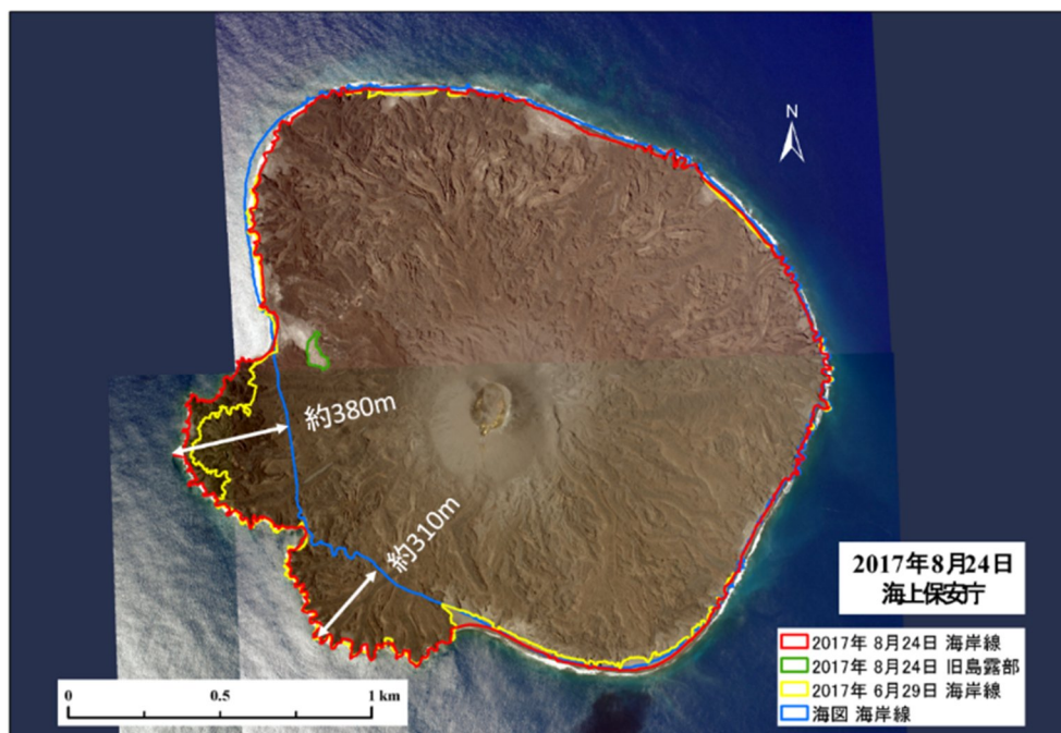
図6 西之島 空中写真（8月24日撮影）
