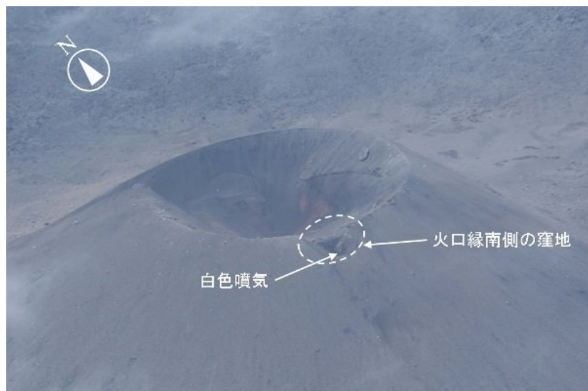
図1 火口縁から放出される白色噴気（8月11日撮影）
