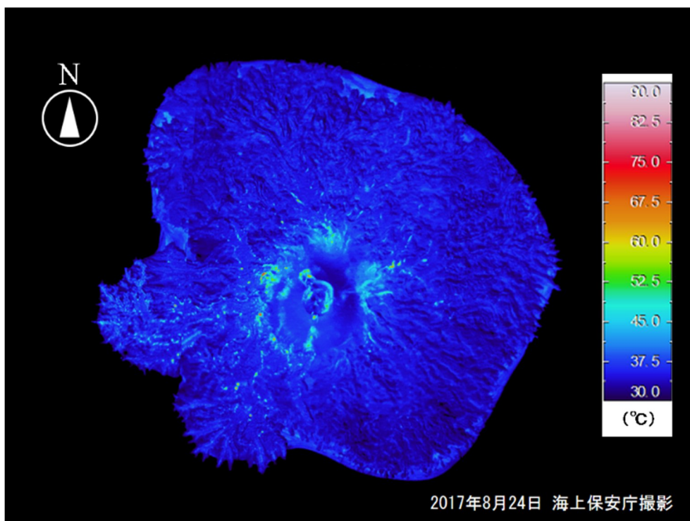
図5 西之島 熱画像（8月24日撮影）
