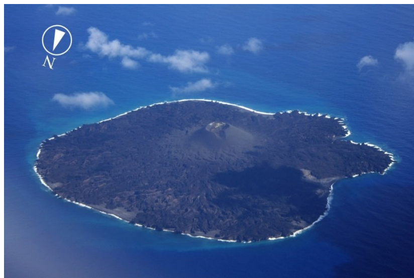
図1 西之島全景（9月13日撮影）
