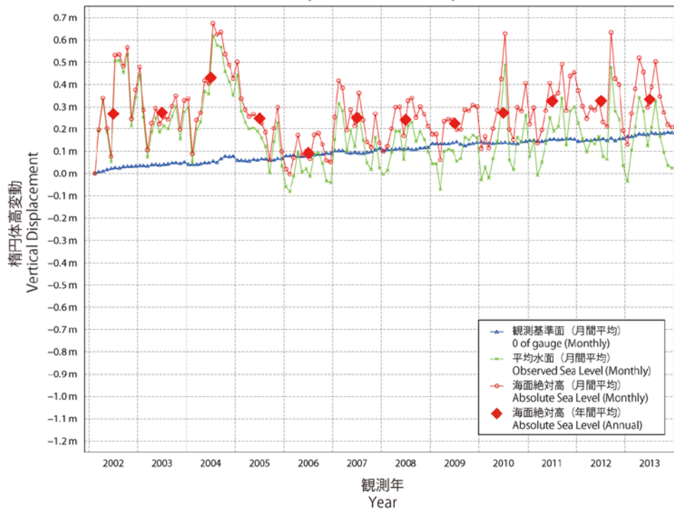
第4図 神津島験潮所の絶対海面高変動
