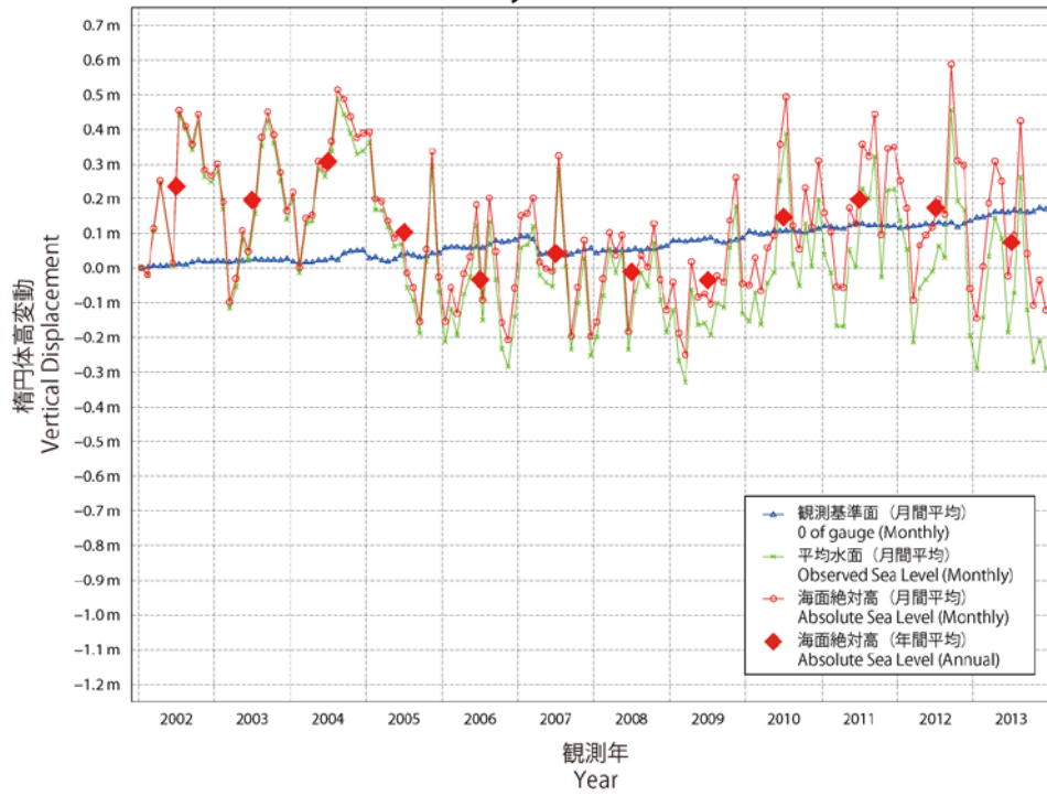
第 5 図 三宅島験潮所の絶対海面高変動
