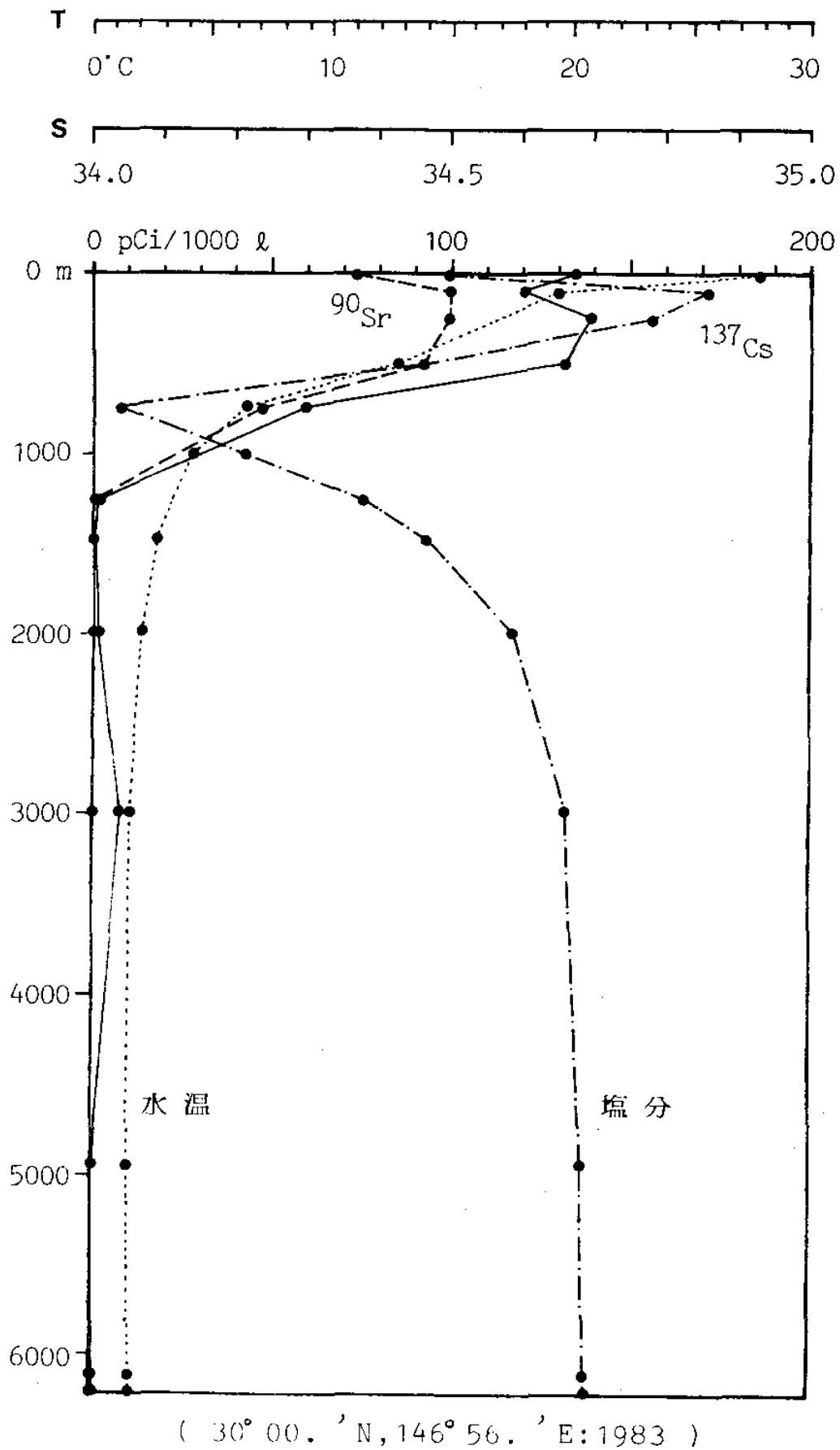
図 26 試験的海洋投棄候補海域 (B海域) における海水中的 Sr-90, Cs-137 および水温, 塩分の鉛直分布
