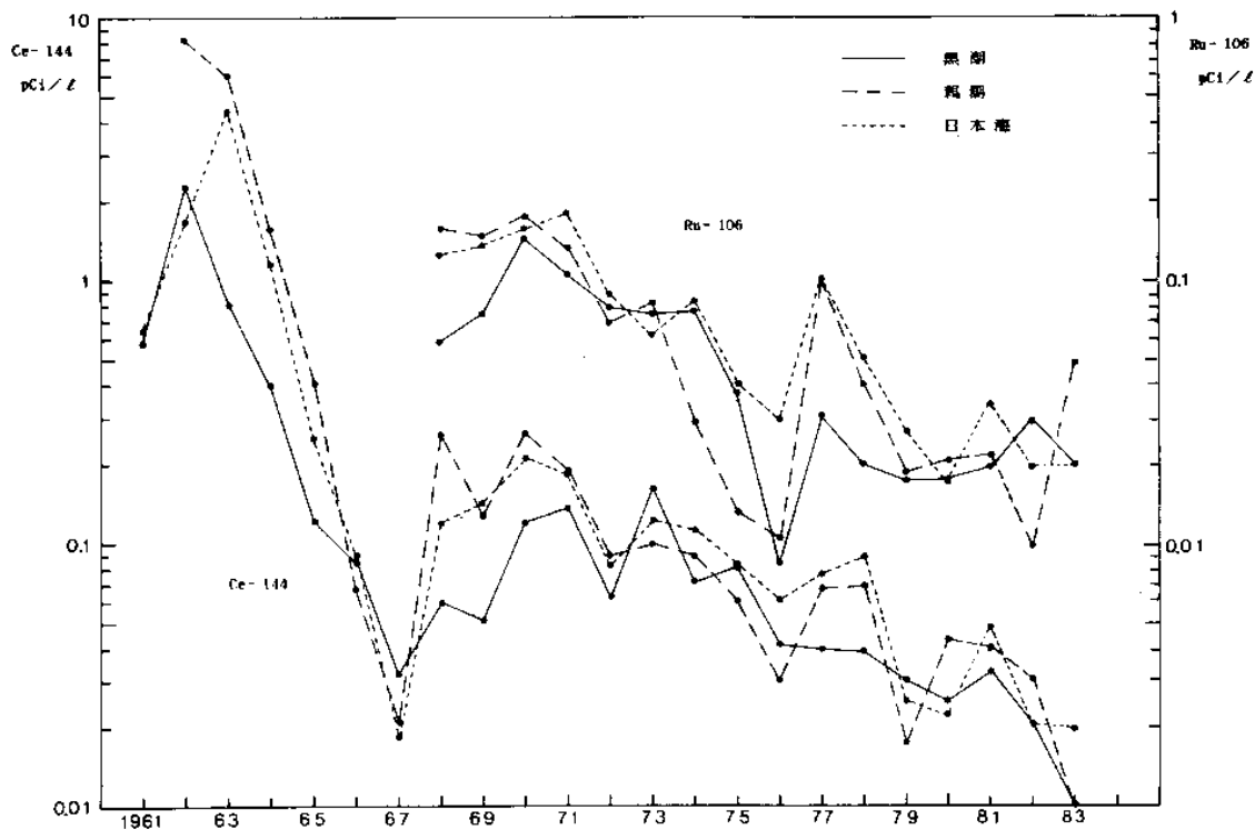
図 7 日本周辺海域表面海水中のCe-144およびRu-106の年平均濃度の経年変化 Fig. 7 Temporal Variation of Yearly Mean Concentrations of Ce-144 and Ru-106 in Surface Sea Water
