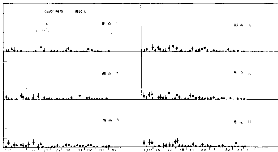
図 22 金武中城港海底土中のCo-60の経年変化
