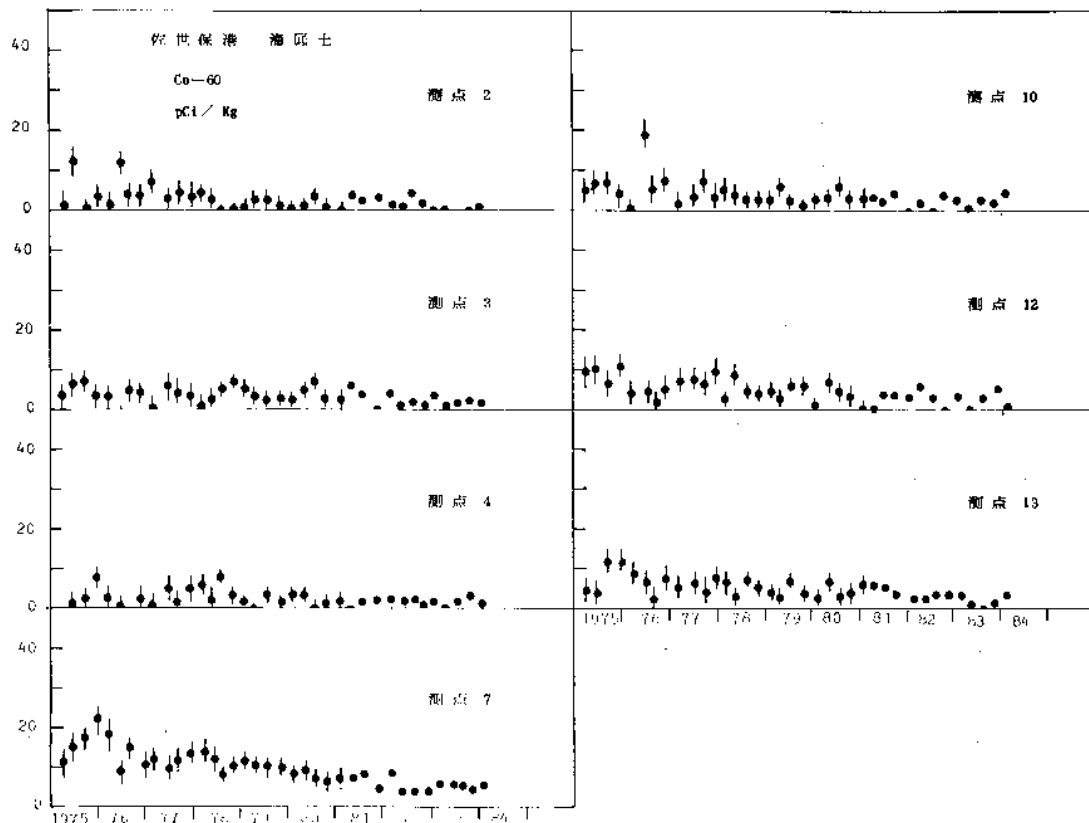
図 21 佐世保港海底土中のCo-60の経年変化
