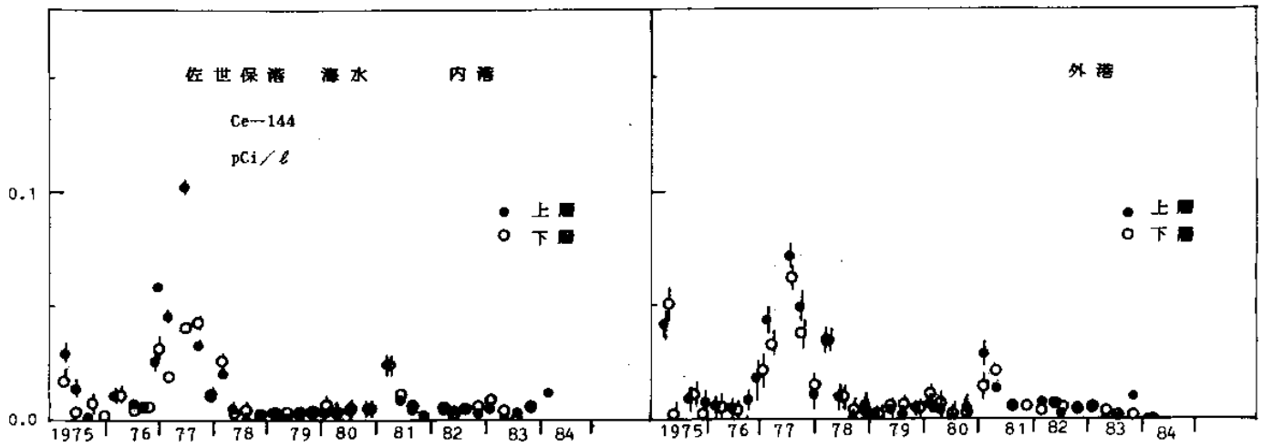
図 16 佐世保港海水中的Ce-144の経年変化
