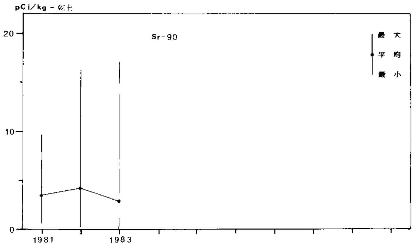
図 12 日本周辺海域海底土中のSr-90の経年変化
