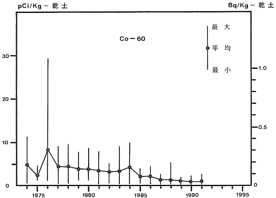
図 1-6 日本近海海底土中の Co-60 の経年変化
