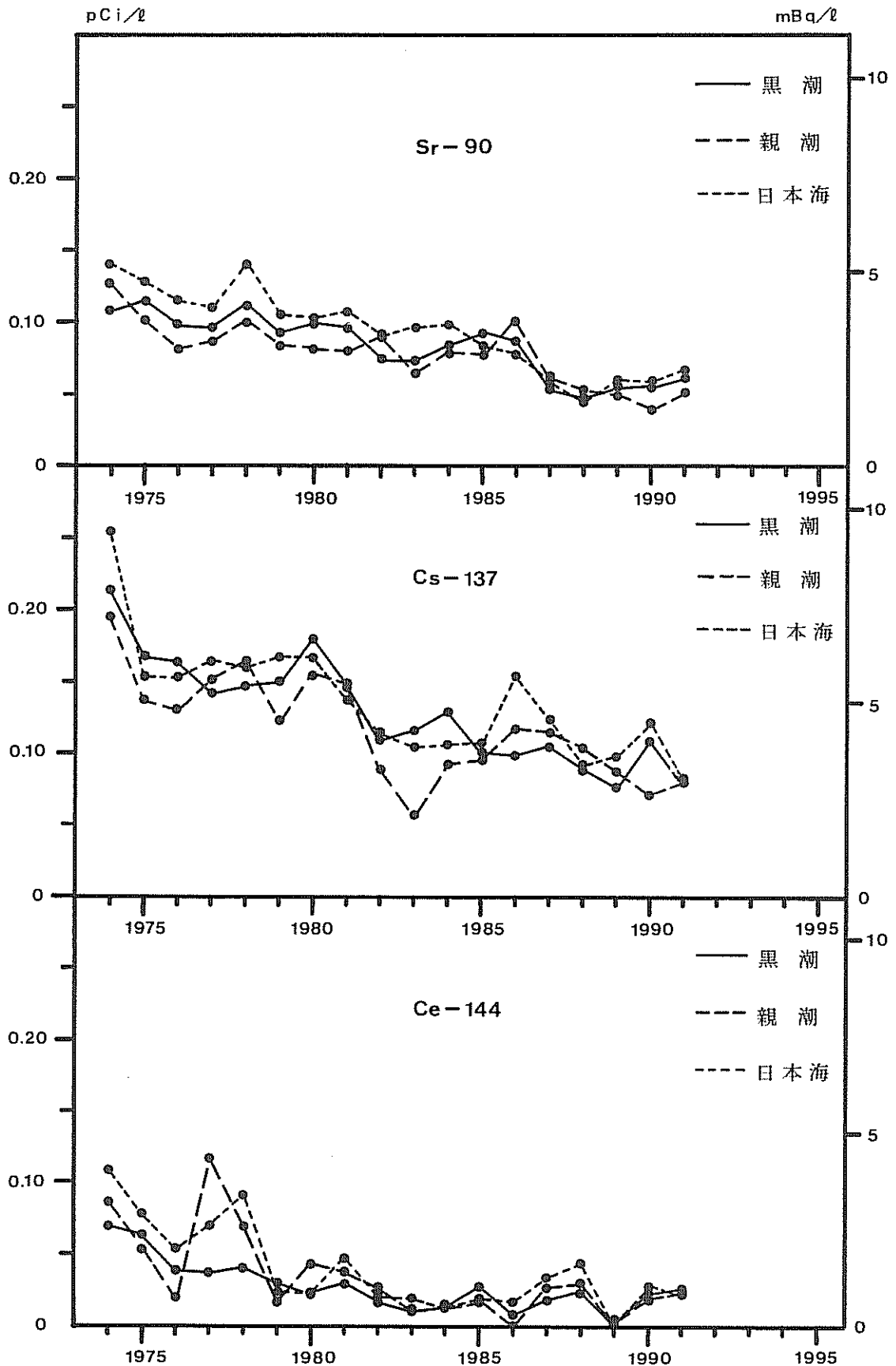
図 1-2 日本近海表面海水中的 Sr-90、Cs-137 及び Ce-144 の年平均濃度の経年変化
