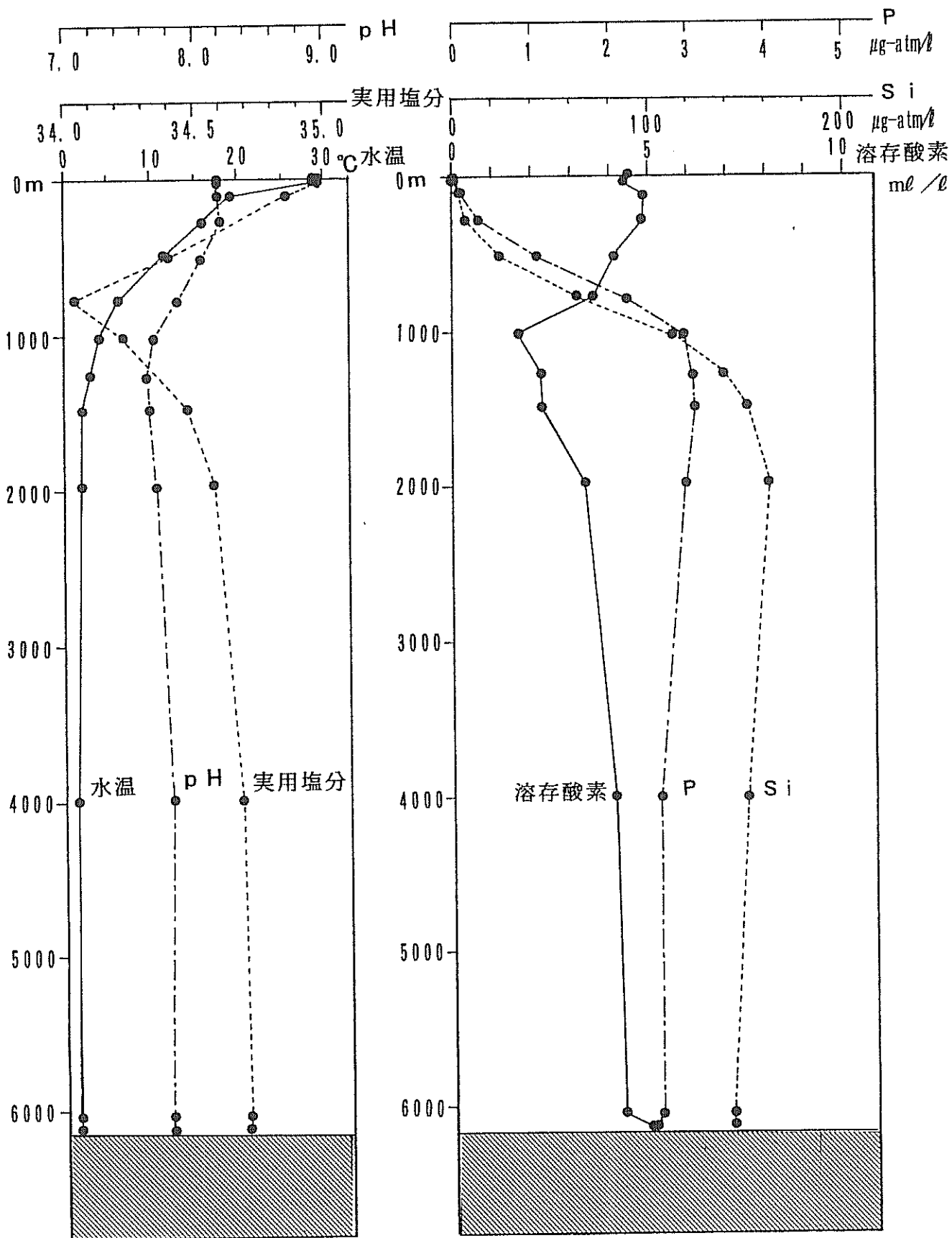
図3-3 測点6 (30°00.0'N, 147°00.0'E) における海水中の水温、実用塩分、溶存酸素、pH、りん酸塩(P)及びけい酸塩(Si)の鉛直分布
