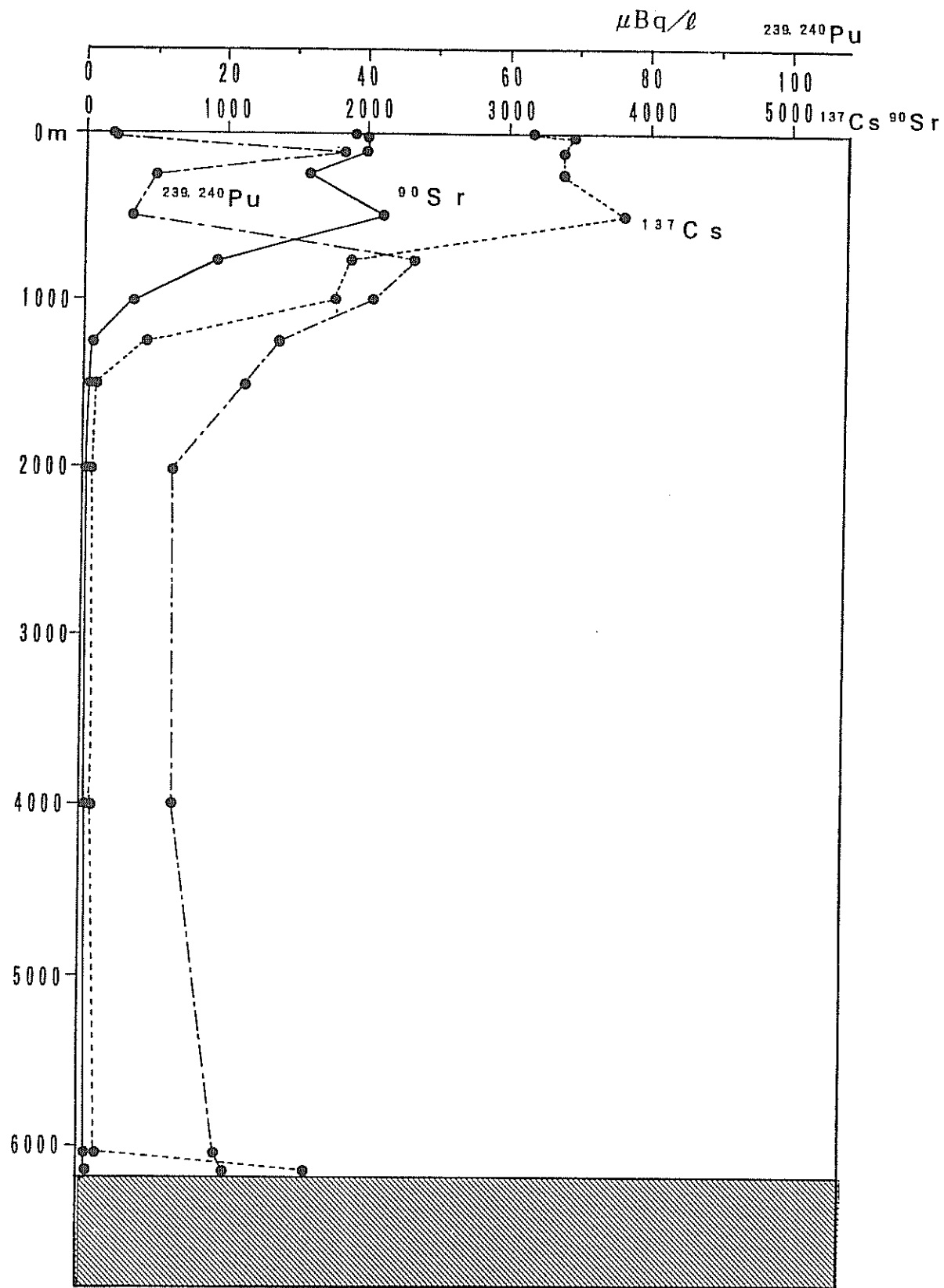
図3-2 測点6 (30°00.0'N, 147°00.0'E) における海水中のPu-239,240、Cs-137及びSr-90の鉛直分布
