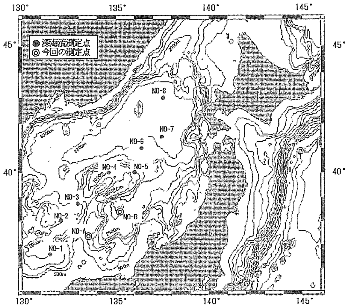
図3-12 深海流速計の測定点
