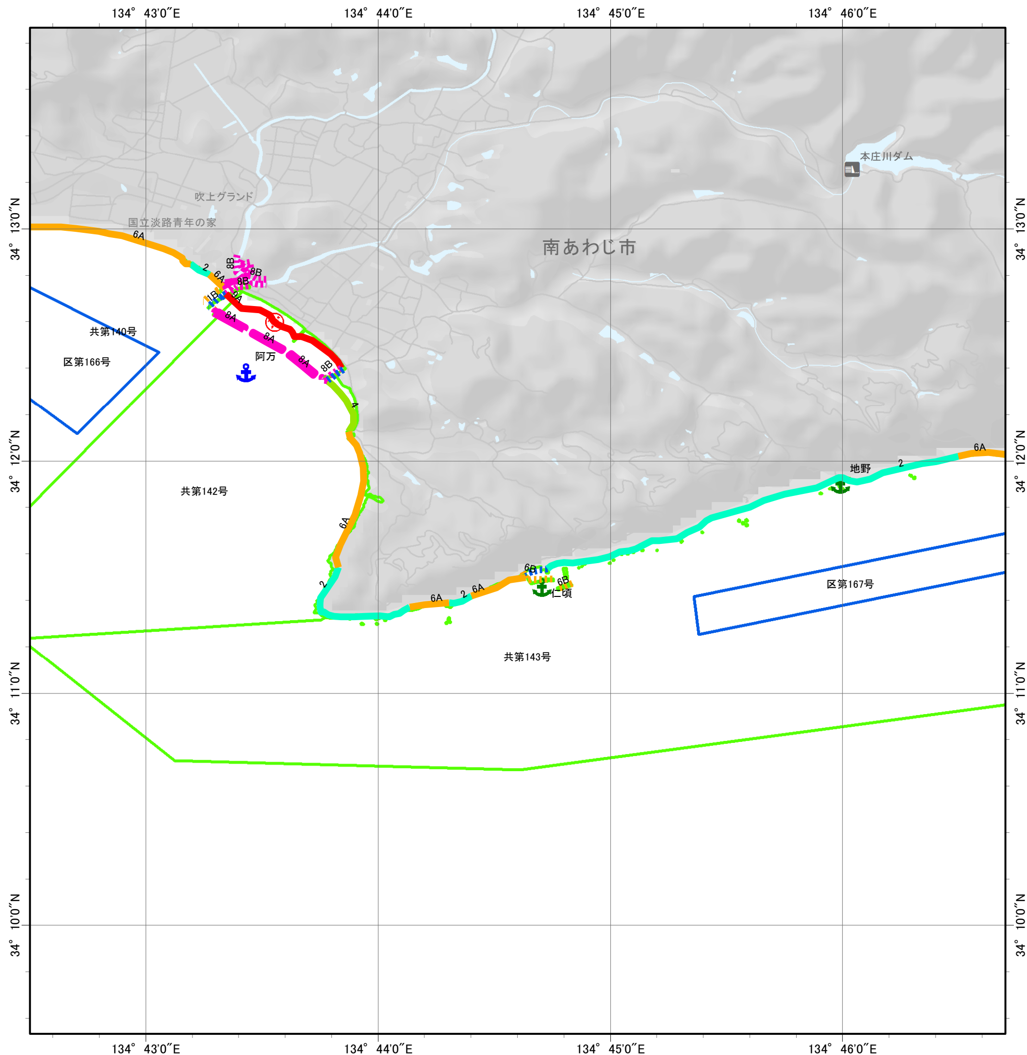
索引図
