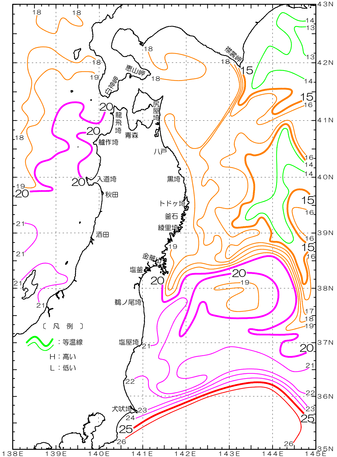
【表面水温水平分布図 (°C)】2006/9/22-10/12
