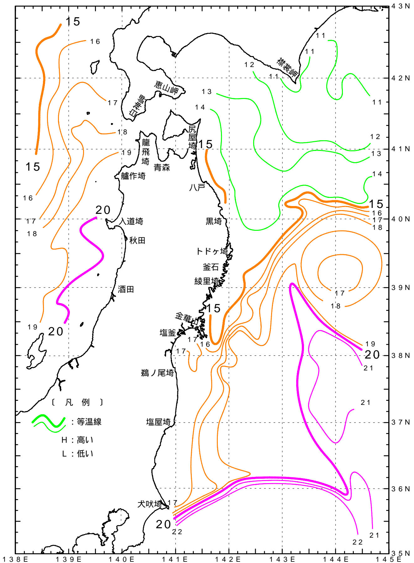
【表面水温水平分布図 ( )】 2008 / 6 / 13 - 6 / 27
