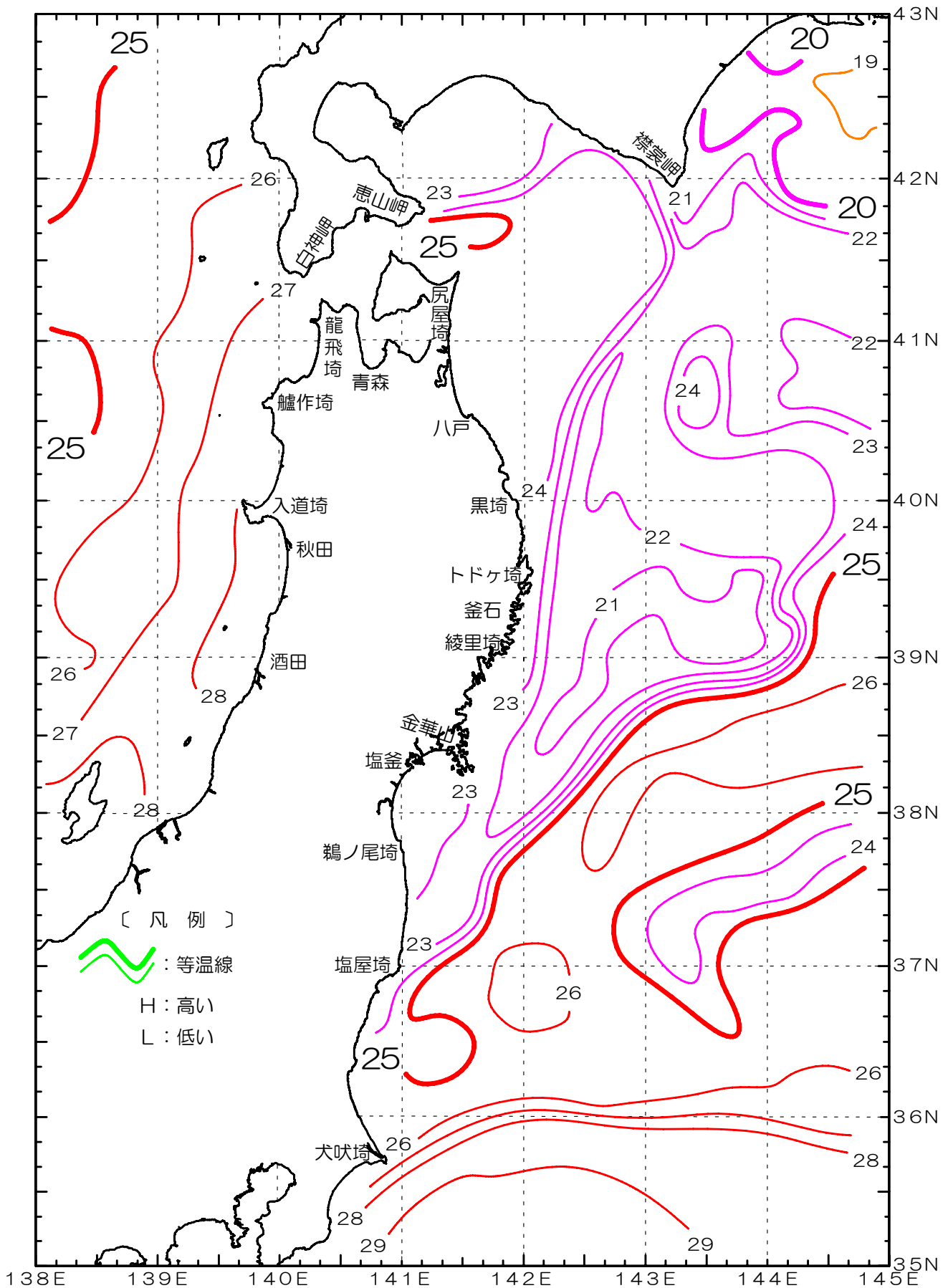
【表面水温水平分布図 (°C)】 2010/9/3-9/16
