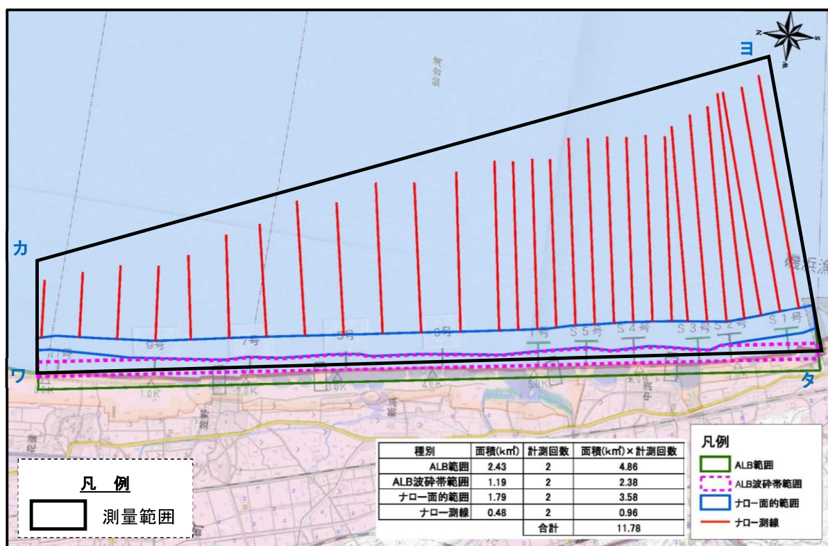
図 4 山元海岸地区(仙台港南部海岸内)
