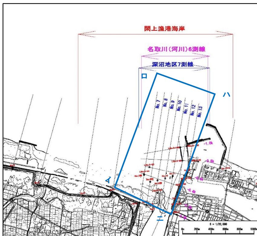
図 2 閑上漁港海岸閑上地区（名取川河口）
