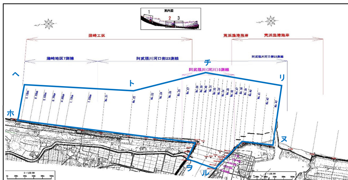
図 3 岩沼海岸納谷地区～荒浜漁港海岸地区（阿武隈川河口）
