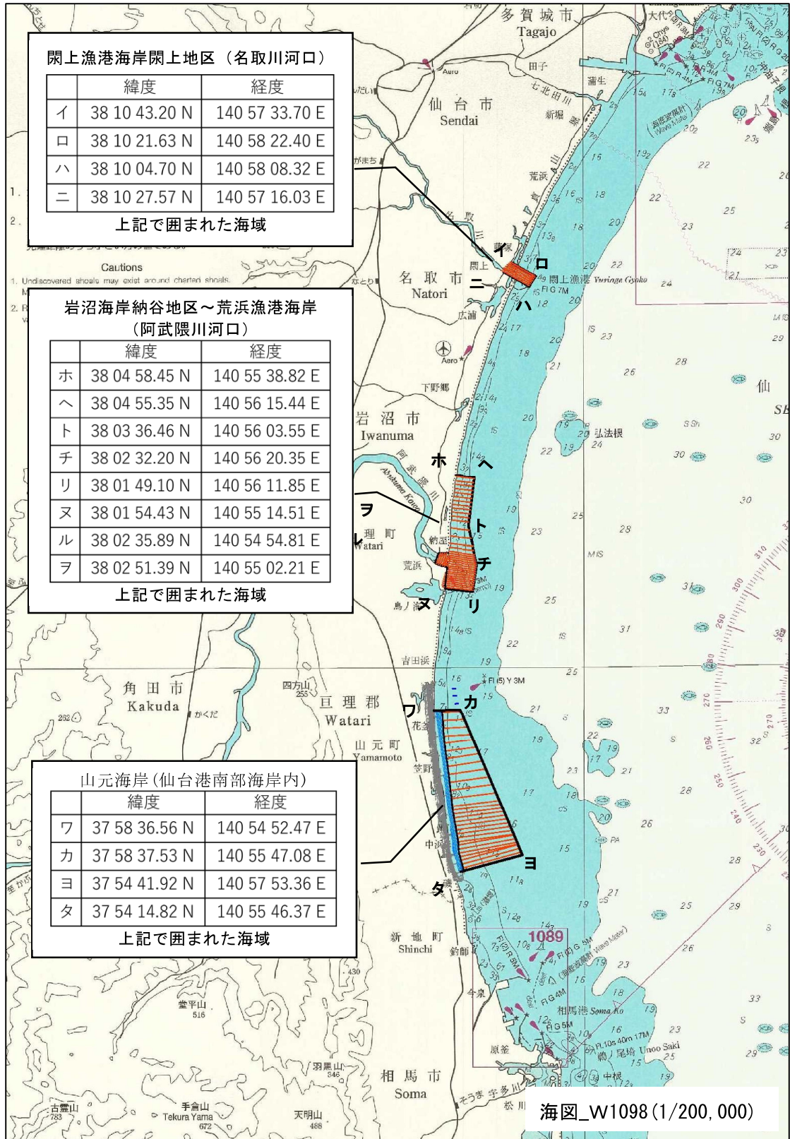
図 1 測量範囲図(全体)
