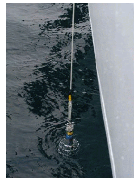
メモリー型STDによる 海底下までの水温・塩 分を測定
