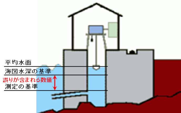
験潮所模式図
