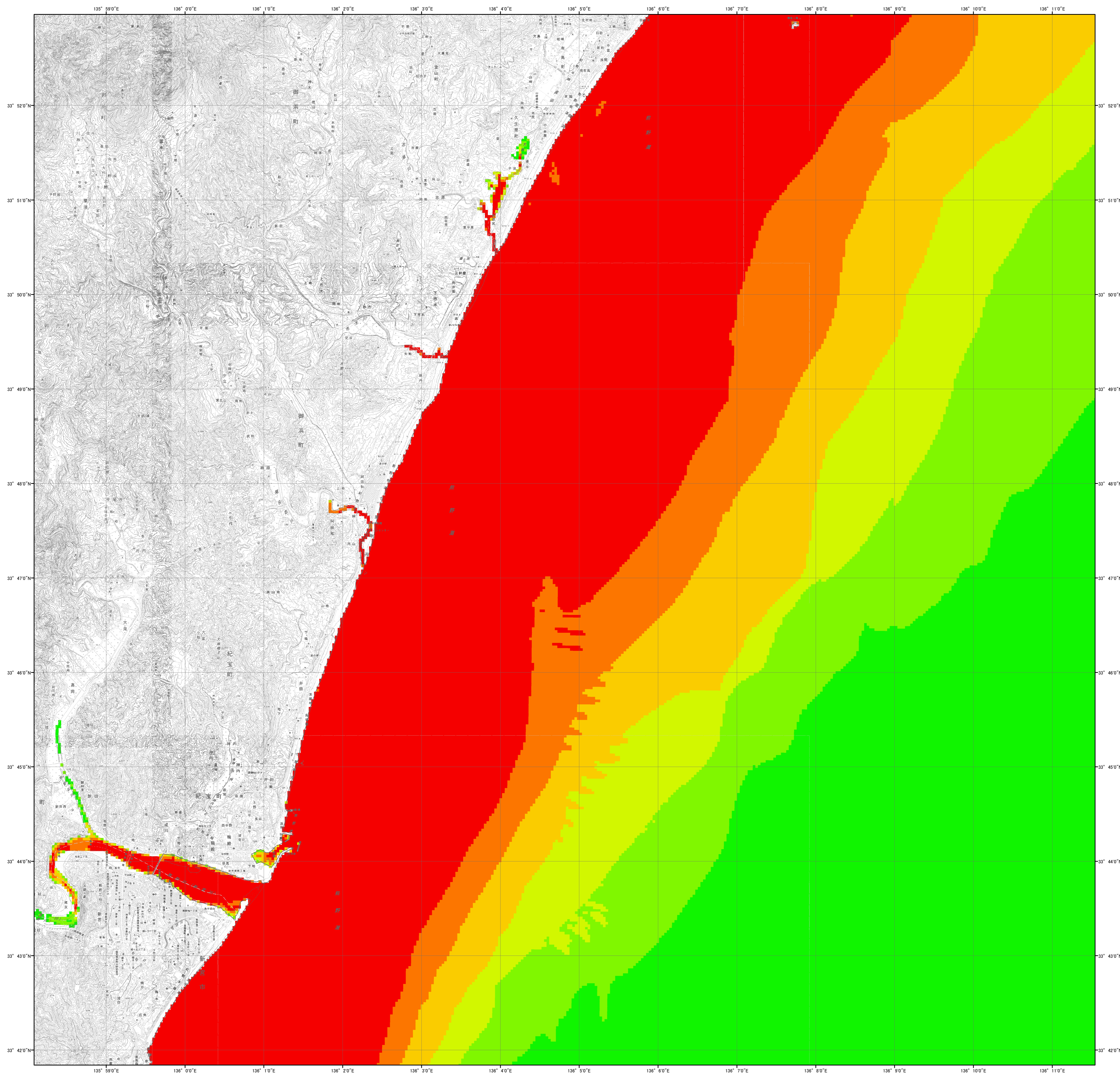
断層モデル
