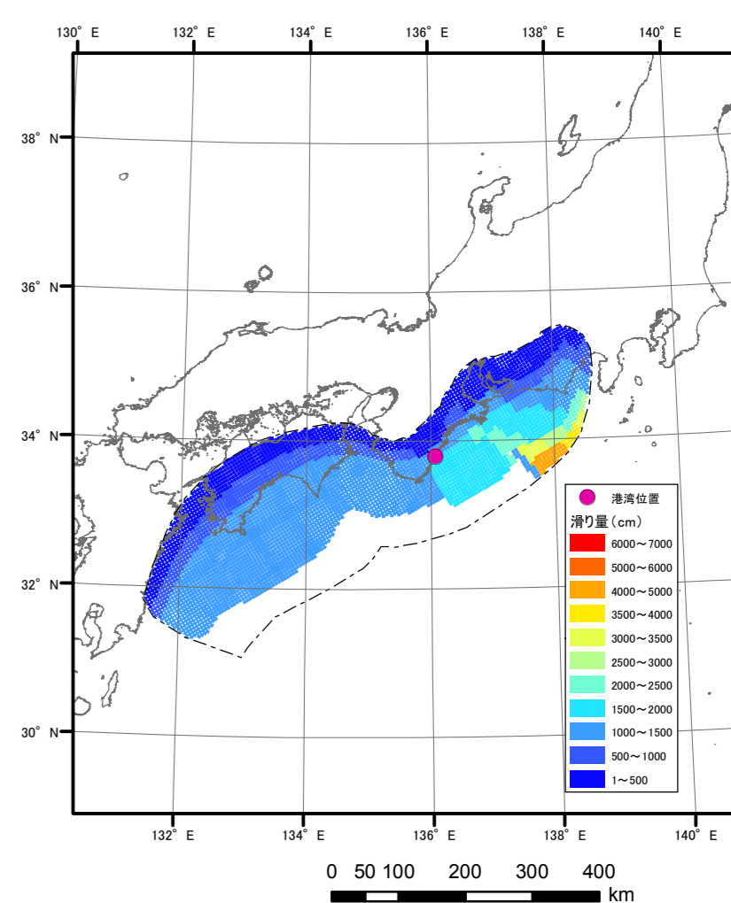
ケース⑥「駿河湾～紀伊半島沖に『大すべり域+（超大すべり域、分岐断層）』
