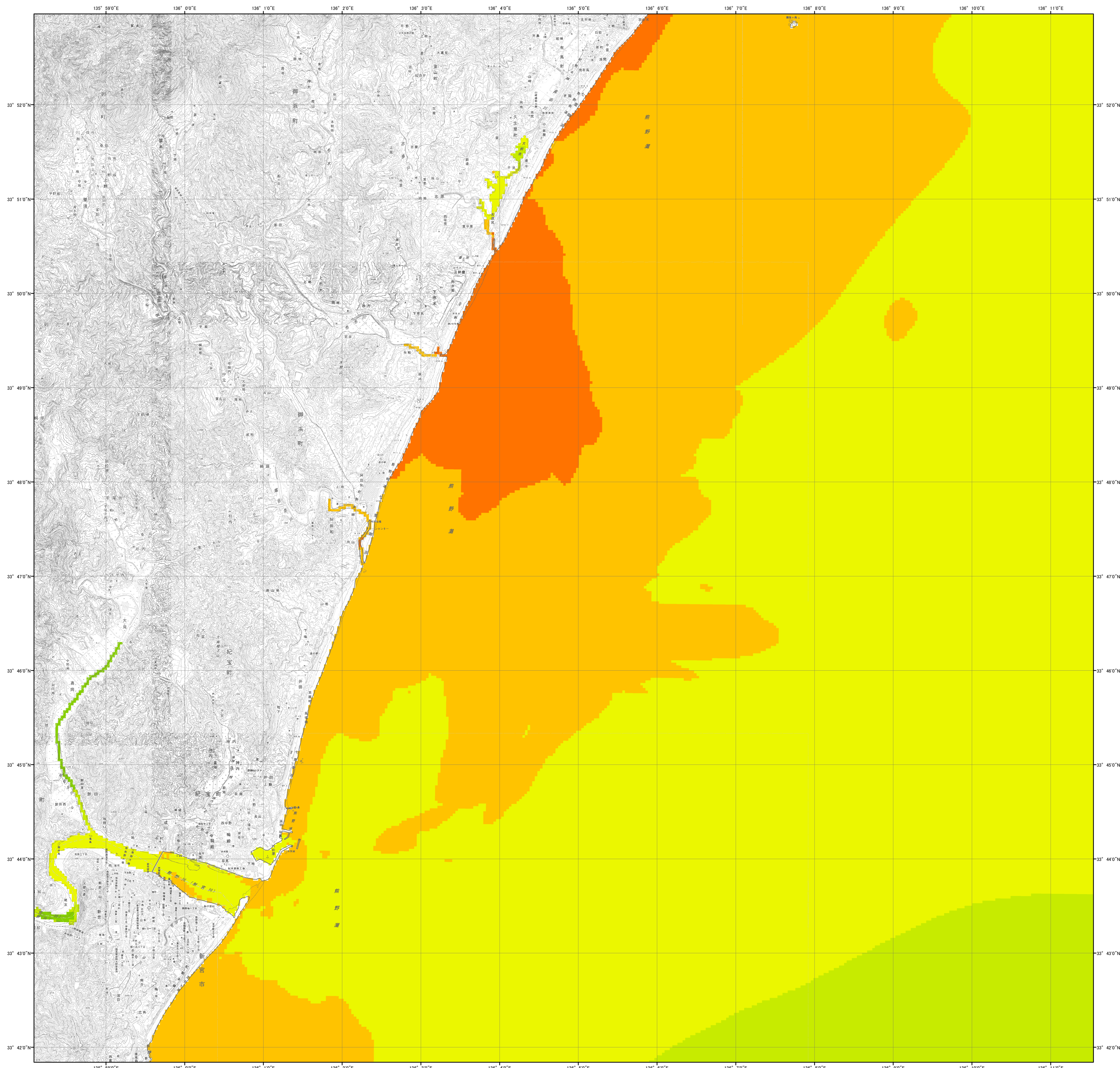
ケース⑥「駿河湾～紀伊半島沖に『大すべり域+（超すべり域、分岐断層）』
