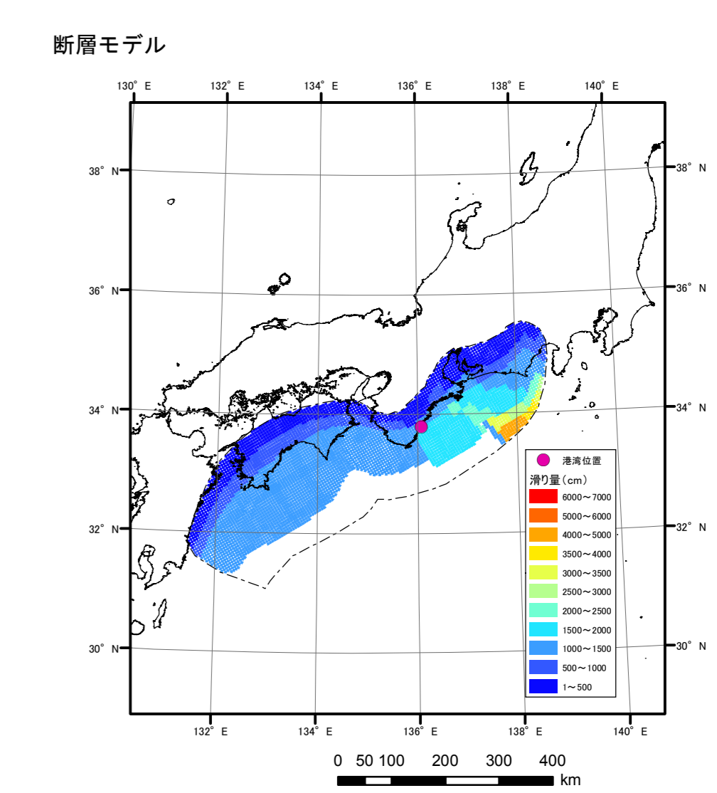
ケース⑥「駿河湾～紀伊半島沖に『大すべり域+（超すべり域、分岐断層）』
