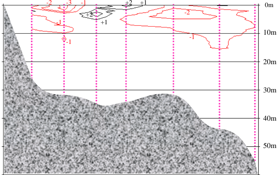
6月22日-15日 塩分変化鉛直断面図
