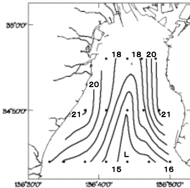
底上水温分布图
