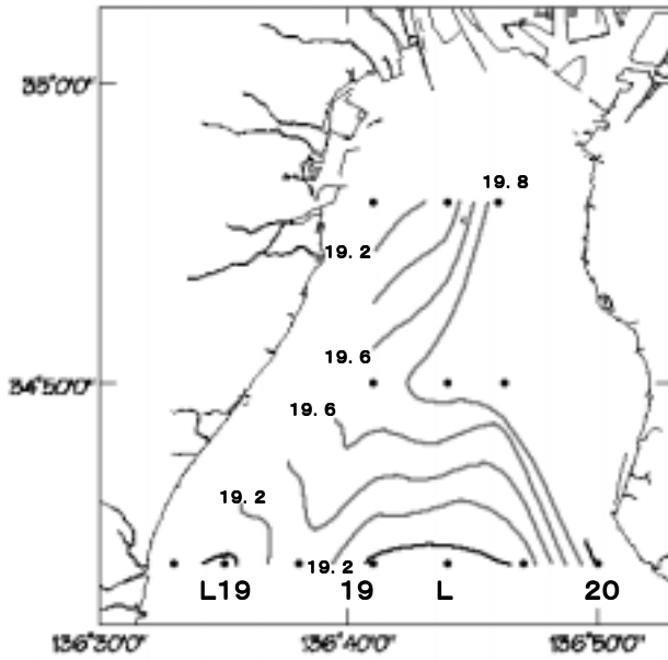
10 m層水温水平分布图
