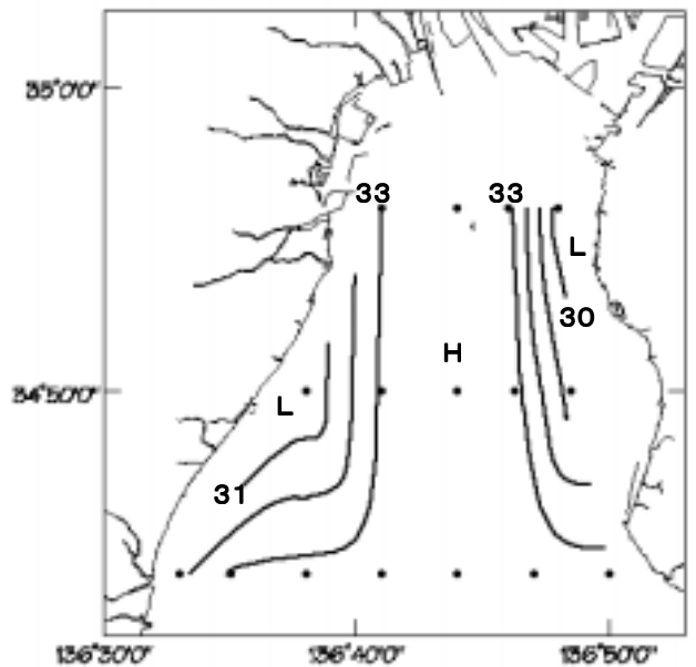
底上塩分分布图
