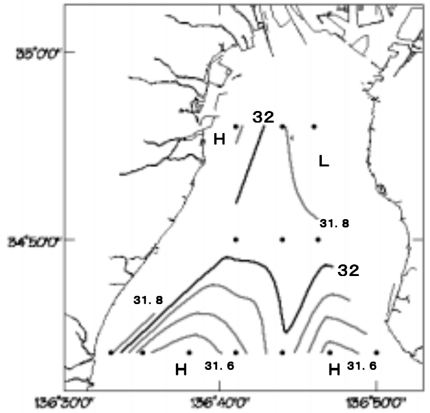
10 m層塩分水平分布图
