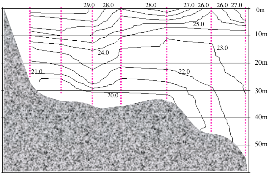
8月22日 水温鉛直断面図
