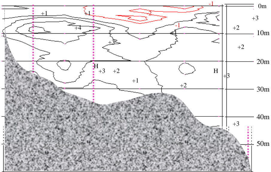
8月22日-11日 水温変化鉛直断面図
