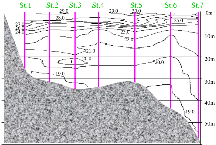
8月11日 水温鉛直断面図
