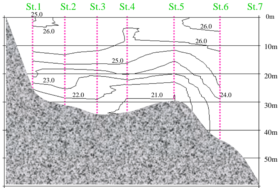
9月13日 水温鉛直断面図
