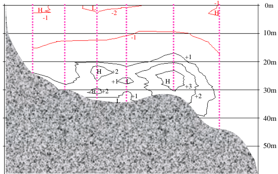
9月27日-13日 水温変化鉛直断面図
