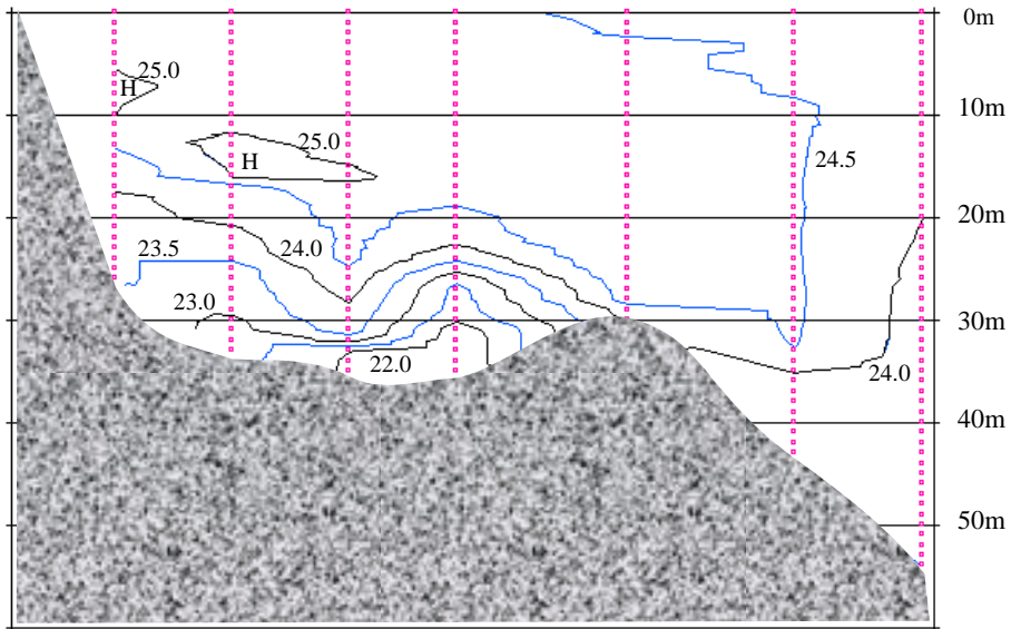
9月27日 水温鉛直断面図
