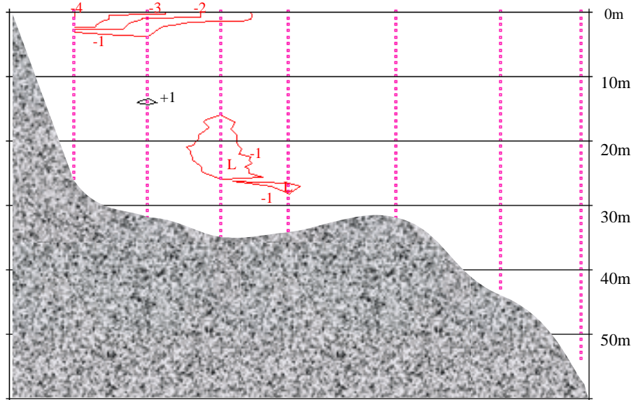
11月27日-13日 塩分変化鉛直断面図
