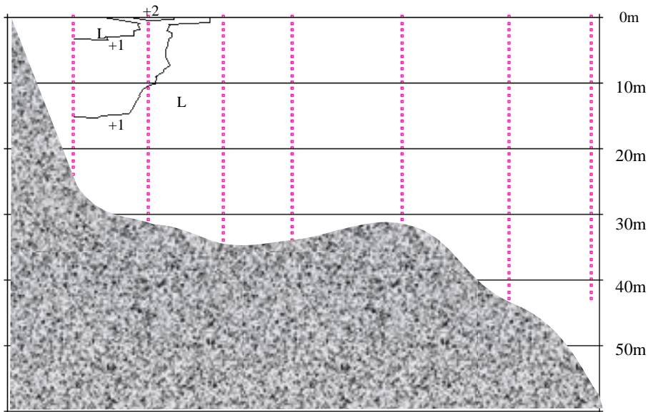
12月27日-9日 塩分変化鉛直断面図
