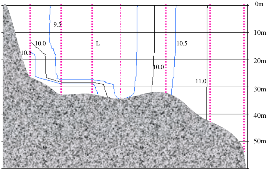
平成13年3月13日 水温鉛直断面図
