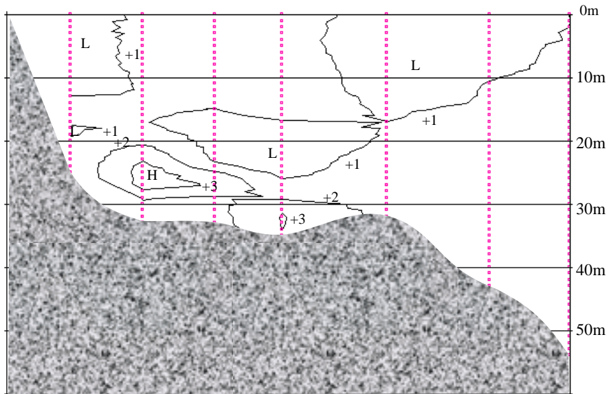
平成13年 3月27日-13日 水温変化鉛直断面図
