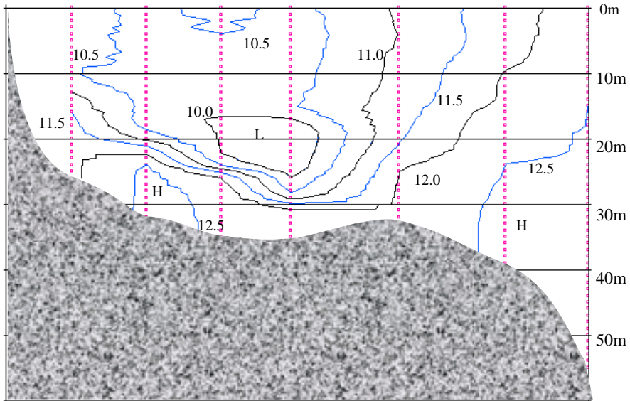
平成13年3月27日 水温鉛直断面図
