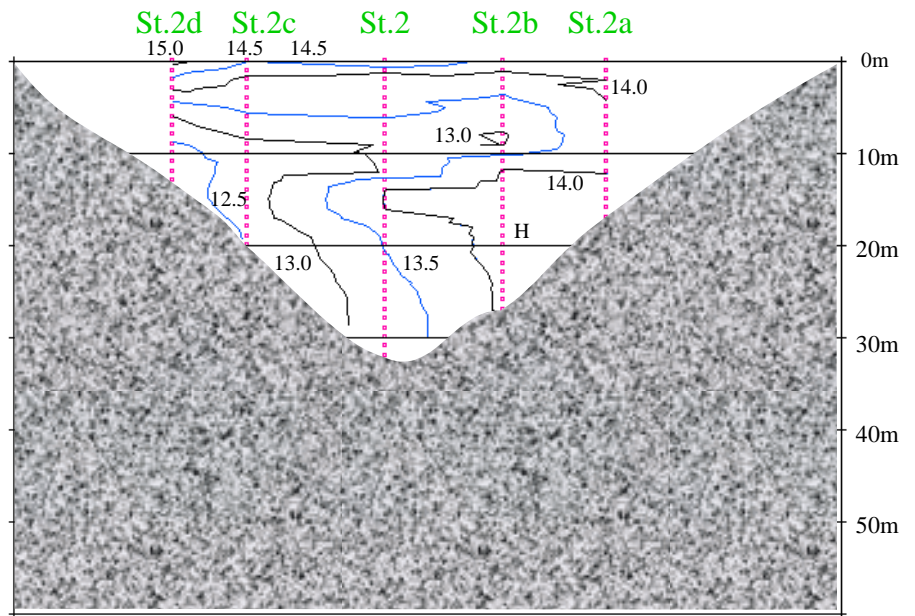
平成13年4月23日 伊勢湾横断測線 水温鉛直断面図
