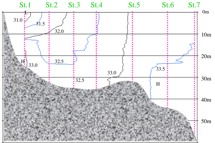
平成13年1月26日 塩分鉛直断面図
