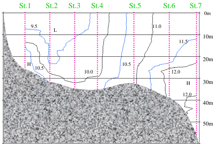
平成13年1月26日 水温鉛直断面図
