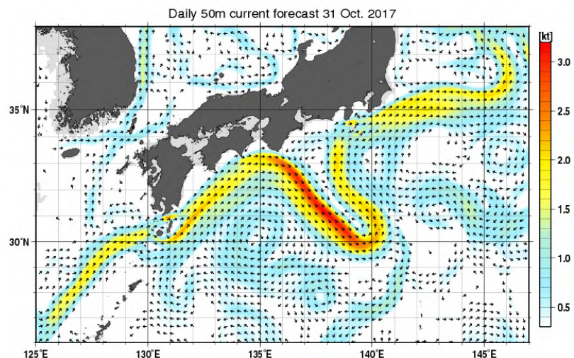
図3 10月31日の深さ50mの海流予測図（気象庁資料）
