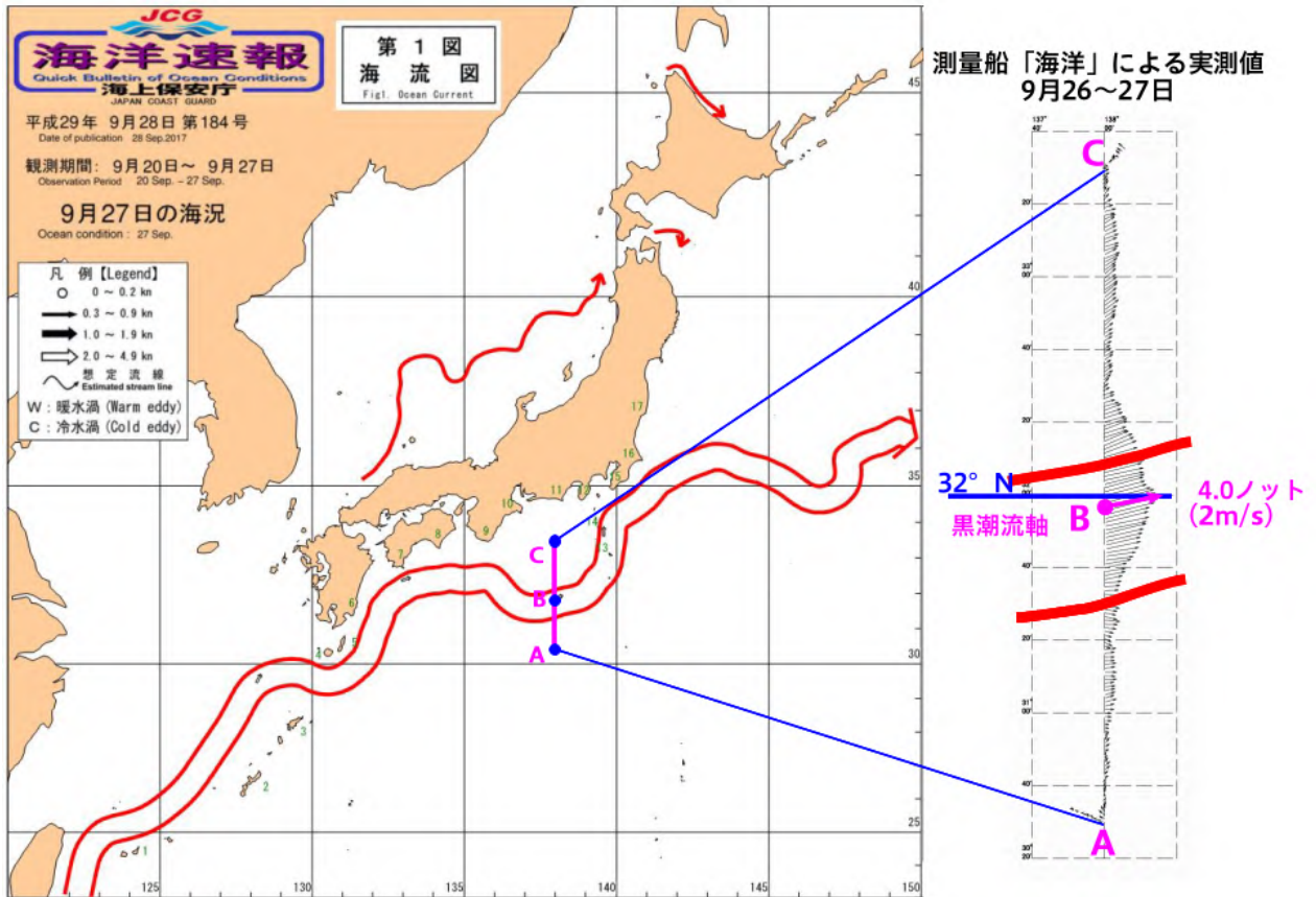
図2 9月27日の海流と測量船「海洋」実測データ（海上保安庁資料）
