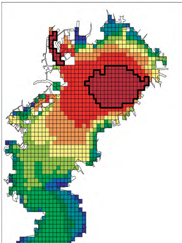
底層DO分布シミュレーション結果 (H24年負荷量・年最低値)
