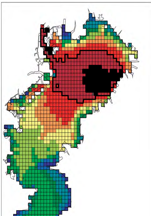
底層DO分布シミュレーション結果 (H16現況負荷量・年最低値)
