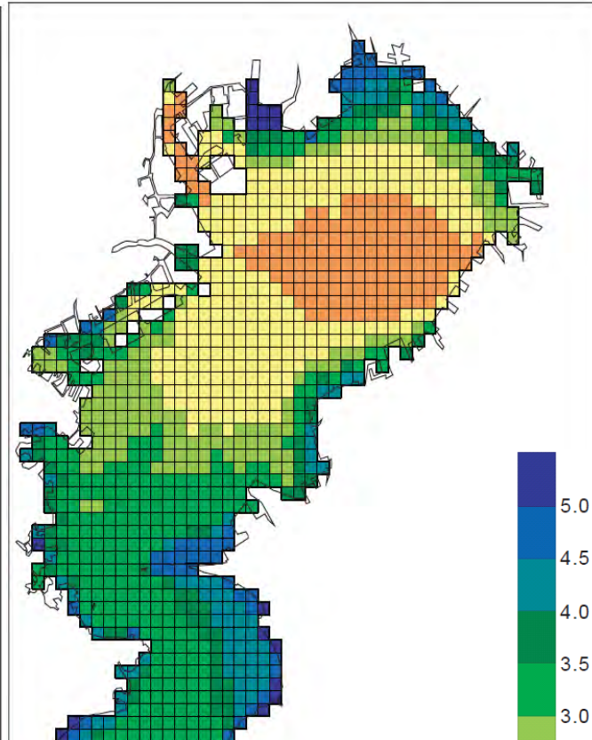
底層DO分布シミュレーション結果 (H36年負荷量・年最低値)
