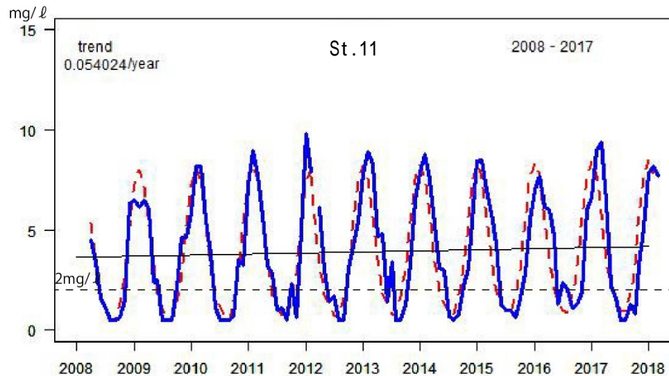
図 B4-2 DO (底層)(mg/L)の時系列変化および重回帰分析結果 (St. 11, 東京都)
