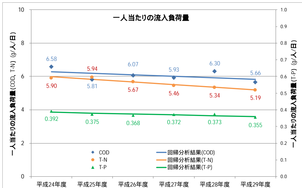
図 D6-3 一人当たりの流入負荷量の回帰分析結果
