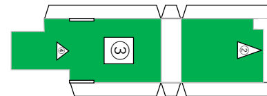
船楼屋根
