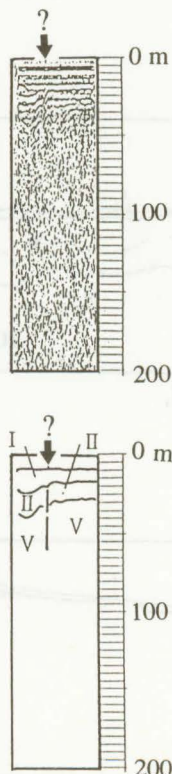
第4図 スーパー音波探査記録例とその解釈図。位置は第1図に示す。
