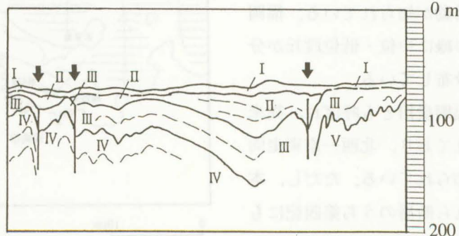
第2図 スパーカー音波探査記録例とその解釈図。位置は第1図に示す。
