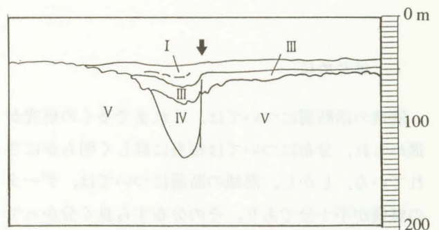
第3図 スパーカー音波探査記録例とその解釈図。位置は第1図に示す。
