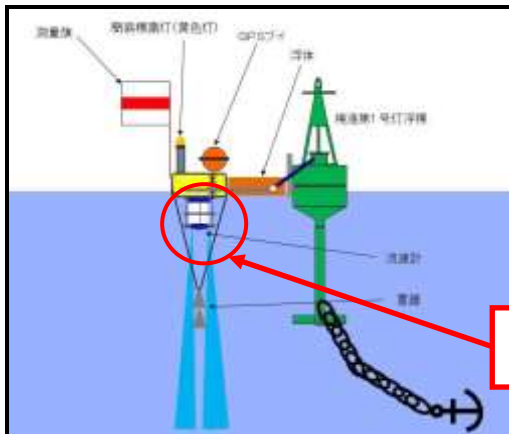
超音波流速計を使用した定点観測
