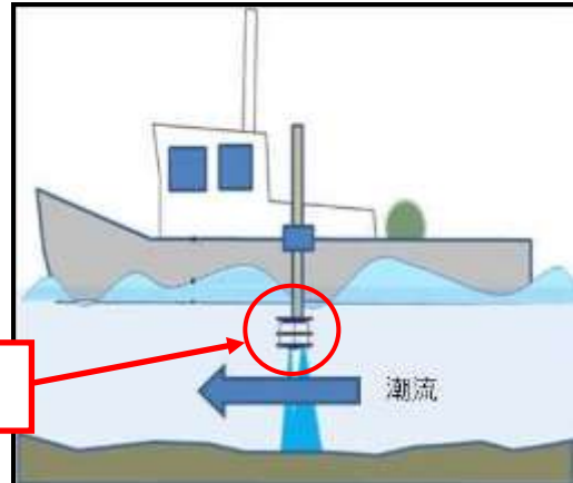
超音波流速計を使用した航走観測
